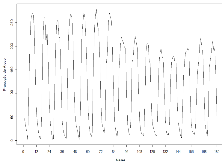
FIGURA 3 - Série de produção brasileira de álcool - índice (média 2002=100), coletada no período mensal de janeiro de 1991 a dezembro de 2005
