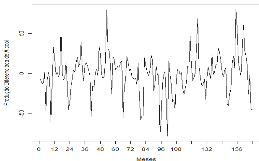
FIGURA 5 - Série de produção brasileira de álcool, em meses, sazonalmente ajustada, no período de janeiro de 1991 a dezembro de 2005
