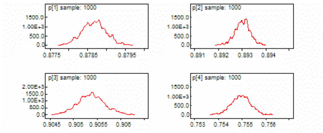
Figura 5 – Distribuição a posteriori de p
