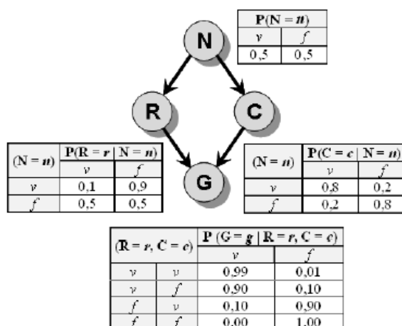
Figura 3 - Rede para a grama molhada citada no Exemplo 2 (MURPHY, 1998)
