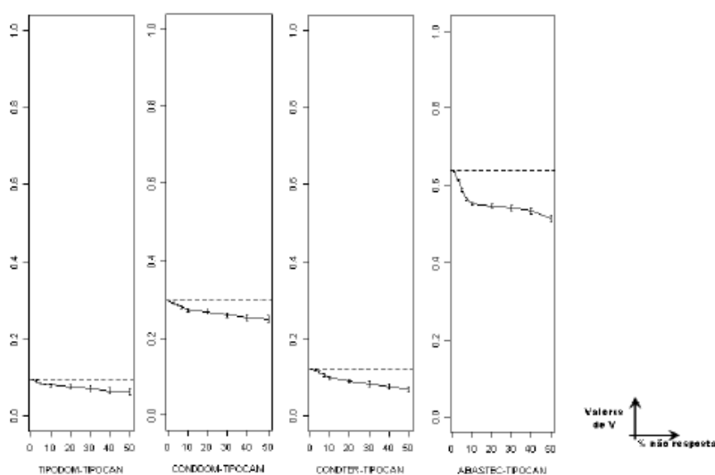
Figura 8 – Gráficos do valor V de Cramer calculado após 500 imputações a partir de rede com cinco nós e em diferentes percentuais de não resposta (a linha tracejada refere-se à medida de associação calculada a partir da base original), dados de Natal, 2000
