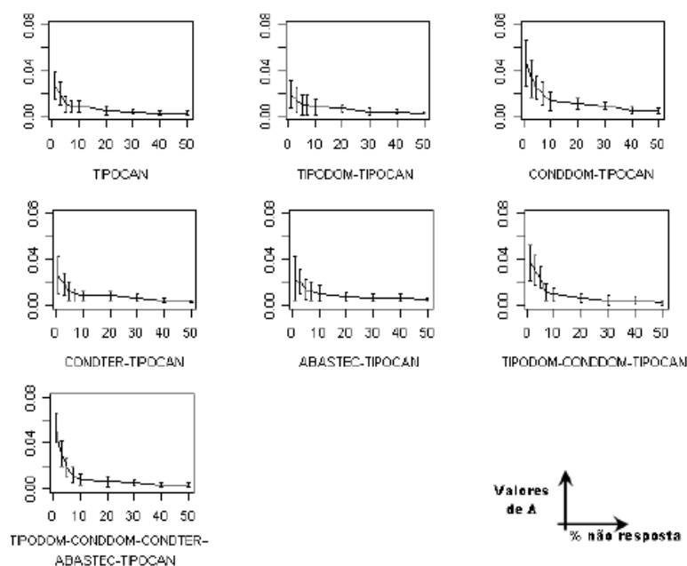
Figura 7 – Resultado da avaliação da consistência estatística – valor de \Delta após 500 imputações a partir de rede com cinco nós e em diferentes percentuais de não resposta, dados de Natal, 2000
