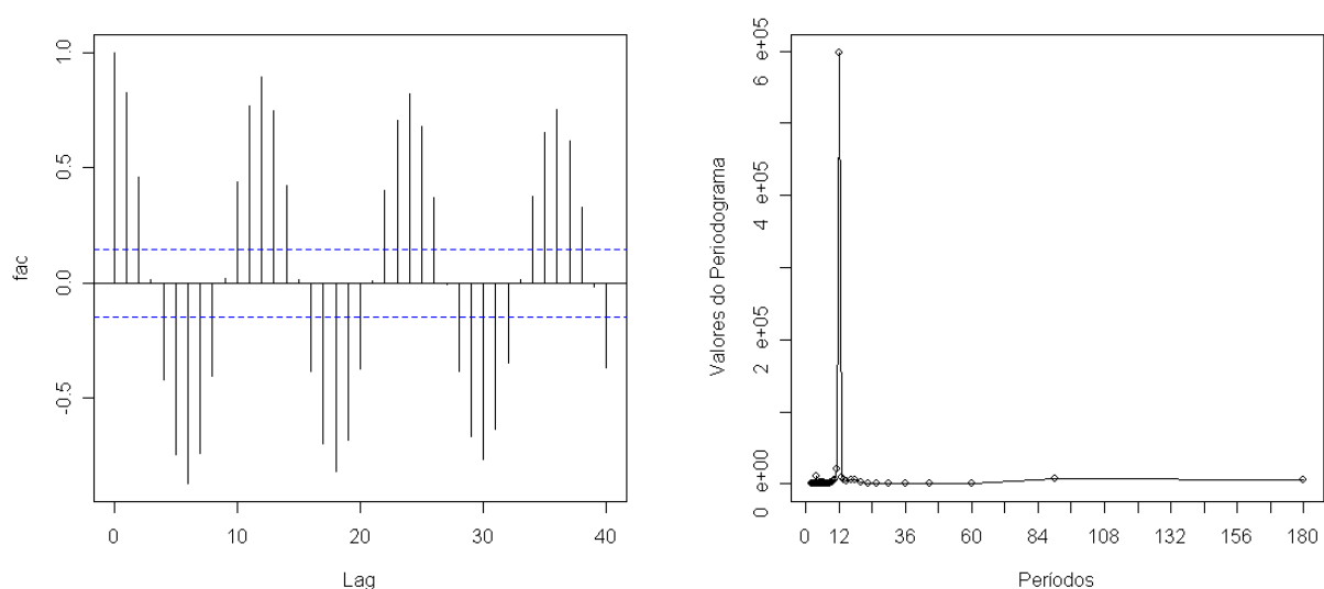
FIGURA 4 - Função de autocorrelação e periodograma da série de produção brasileira de álcool, coletada no período mensal de janeiro de 1991 a dezembro de 2005
