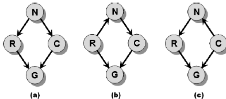
Figura 4 - (a) Rede original (de Murphy, 1998) e (b) e (c) Elementos da classe de equivalência da rede original para o Exemplo 2
