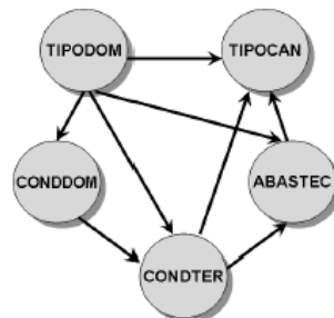
Figura 6 – Grafo da rede ajustada para cinco variáveis discretas
