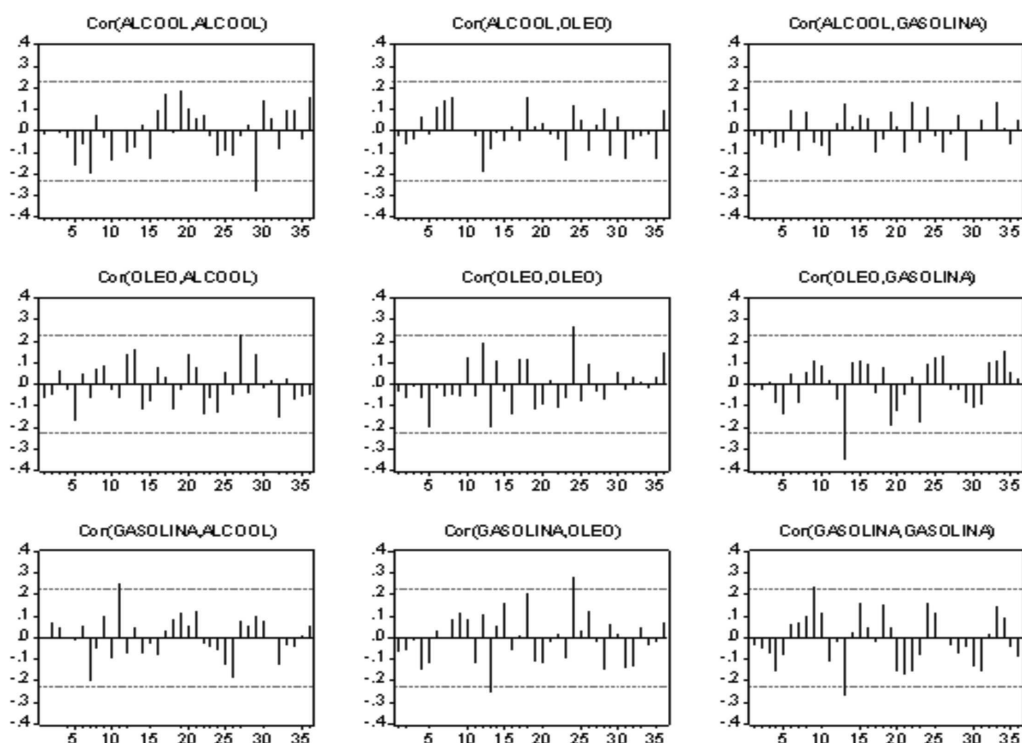
FIGURA 11 - Representação gráfica da função de correlação dos resíduos das produções brasileiras de álcool, óleo diesel e gasolina, em metros cúbicos (m 3 ), no período mensal de janeiro de 2000 a setembro de 2006
