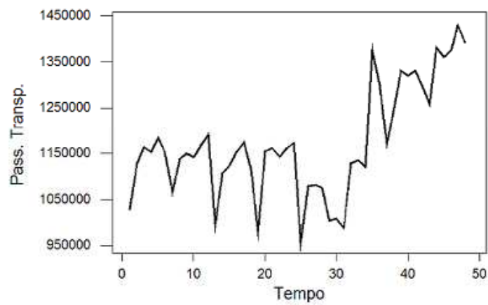
Figura 2 – Série Original – Livre do Efeito Tendência
