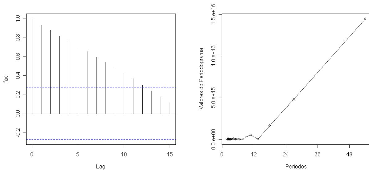
FIGURA 8 - Função de autocorrelação e periodograma da série de produção brasileira de cana-de-açúcar, em milhões de toneladas, no período anual de 1947 a 1998
