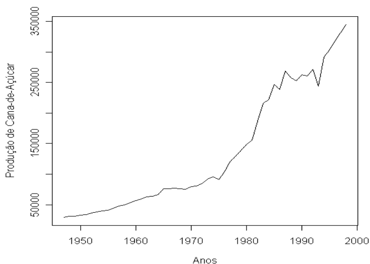
FIGURA 7 - Série de produção brasileira de cana-de-açúcar, em milhões de toneladas, no período anual de 1947 a 1998
