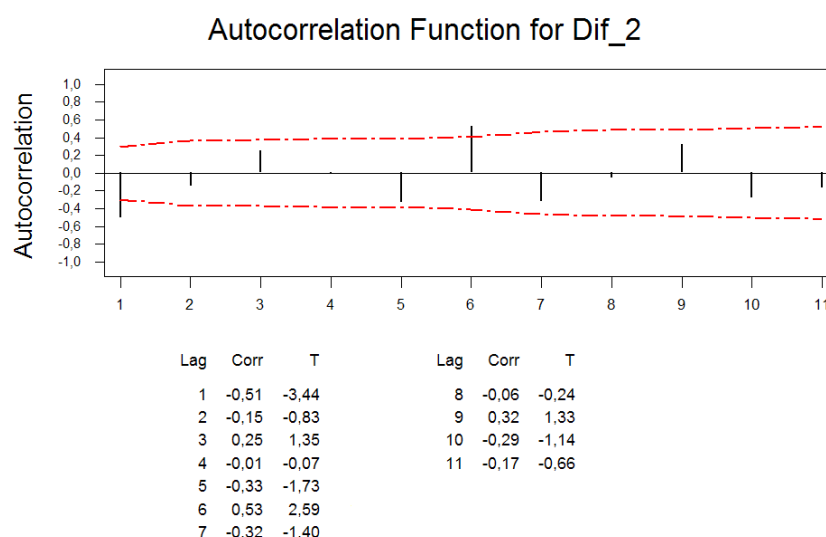
Figura 4 – Correlograma da Série Transformada Y_t
