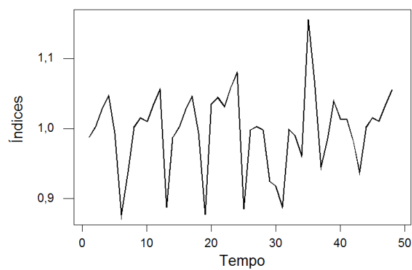
Figura 3 – Série Original e Série Sazonalmente Ajustada
