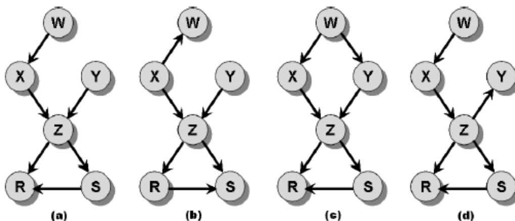
Figura 5 - Exemplo de identificação de elementos de uma mesma classe de equivalência (reproduzido de Neapolitan (2004))
