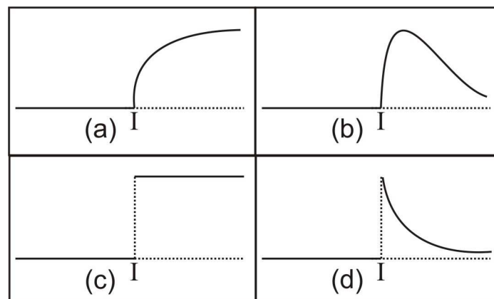
FIGURA 1- Efeito gradual permanente (a), gradual temporário (b), abrupto permanente (c) e abrupto temporário (d), sobre uma série temporal Z_t
