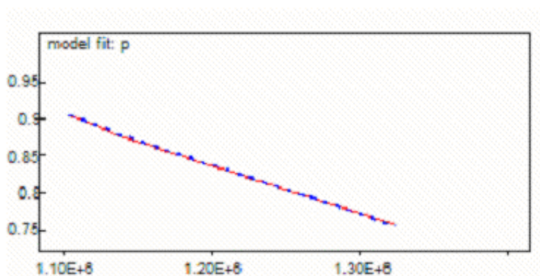
Figura 6 – Valores Ajustados p_i versus Valores Médios da Série Mensal dos Passageiros 2001-2004
