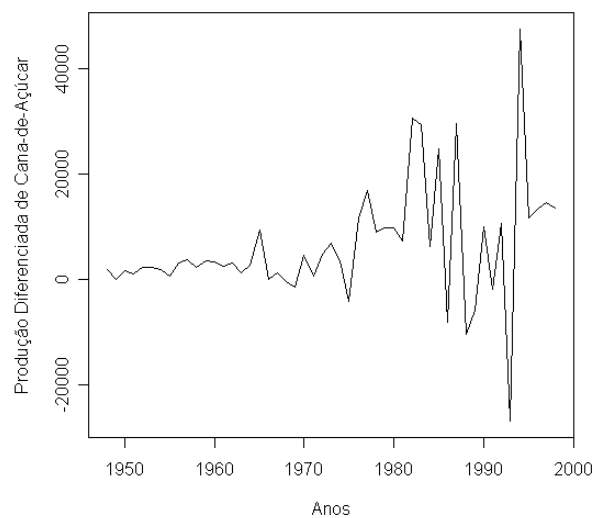
FIGURA 9 - Série diferenciada da produção brasileira de cana-de-açúcar, em milhões de toneladas, no período anual de 1947 a 1998
