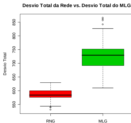
Figura 4.3 - Gráfico comparativo do comportamento do Desvio Total entre a RNG e o MLG referente à base Caranguejo
