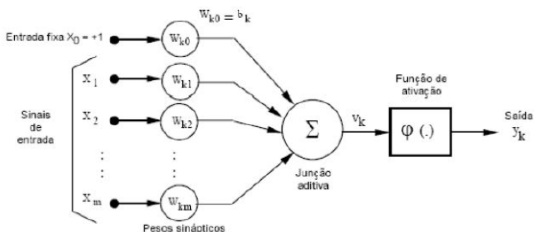
FIGURA 1 - Modelo não linear de um neurônio [Haykin, 2001]
