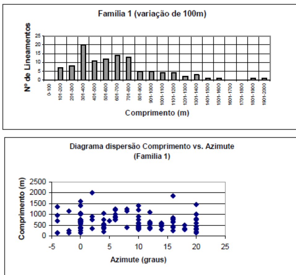
Figura 5 Histograma e diagrama de dispersão Família 1
