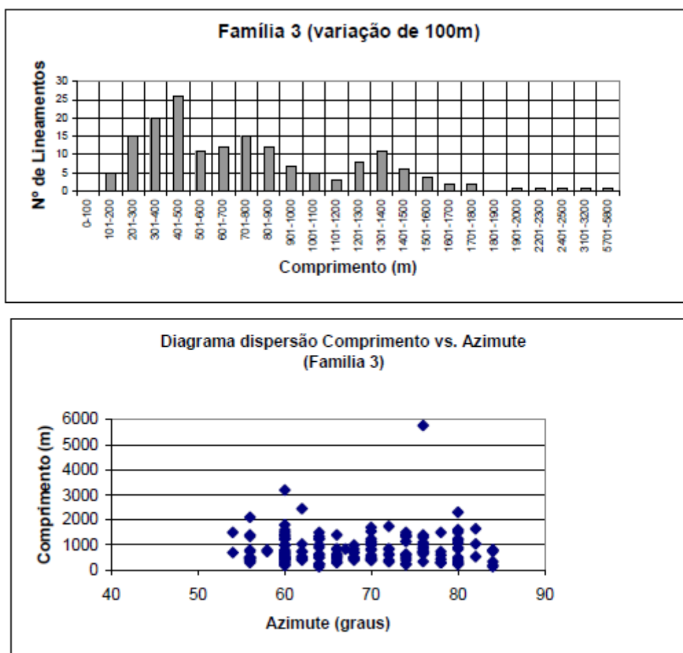
Figura 7 Histograma e diagrama de dispersão Família 3.
