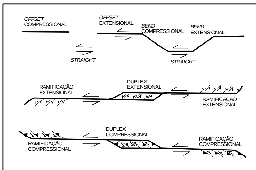
Figura 2. Esquema da geração de duplexes e ramificações, extensionais e compressionais, em um sistema de zona de cisalhamento transcorrente levógiro (modificado de Woodcock e Fischer, 1986).
