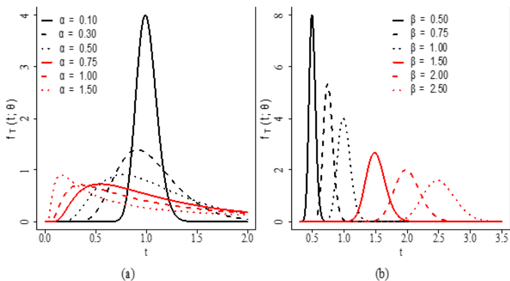
Figura 1: Gráficos da f.d.p da BS para \beta = 1.0 (a) e \alpha = 0.1 (b)
