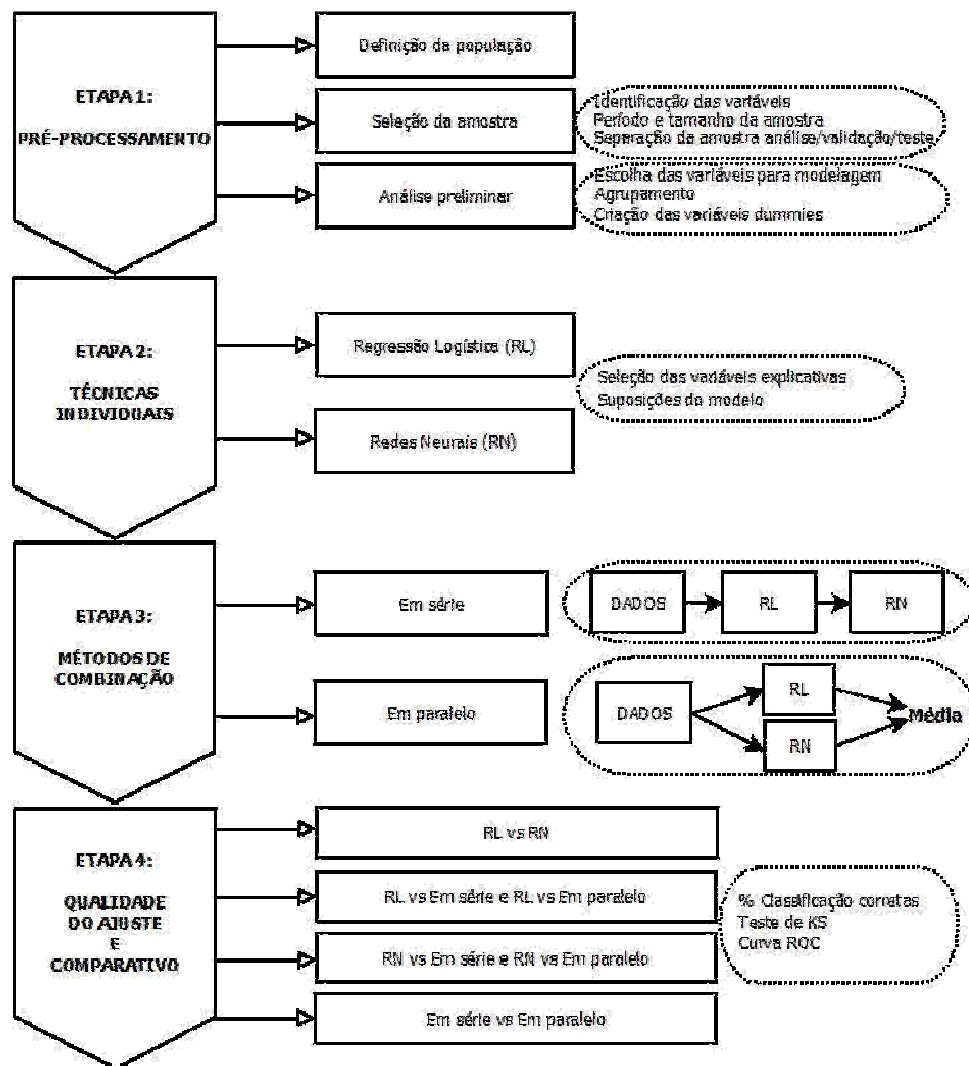
Figura 3 - Método Proposto
