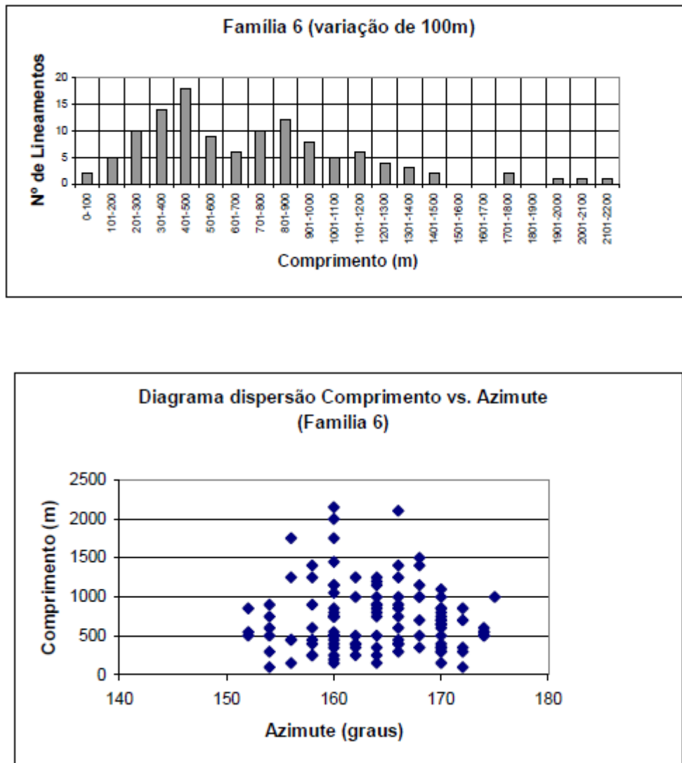
Figura 10 Histograma e diagrama de dispersão Família 6.
