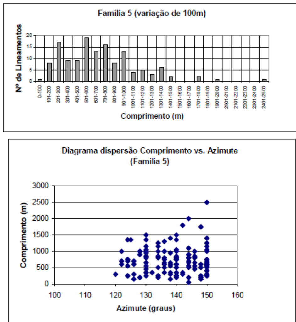
Figura 9 Histograma e diagrama de dispersão Família 5
