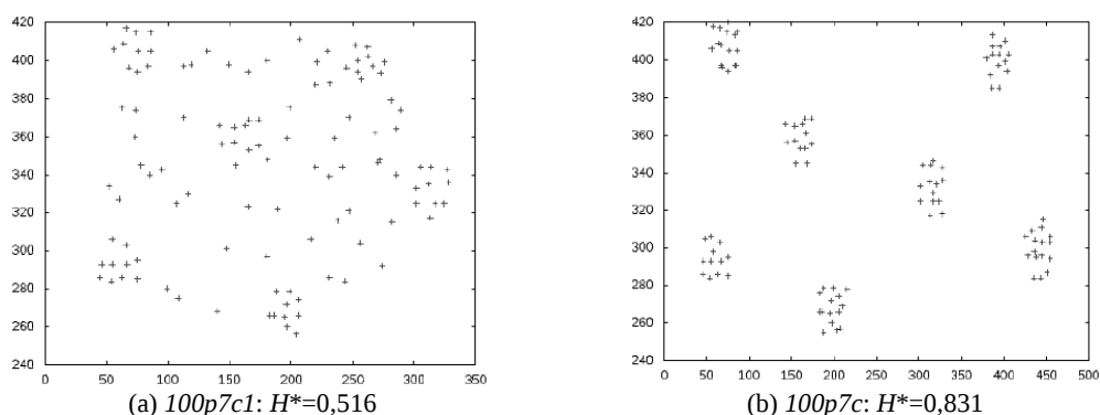
Figura 3: Instâncias 100p7c1 e 100p7c. H^* é a mediana dos valores H em 1000 iterações.
