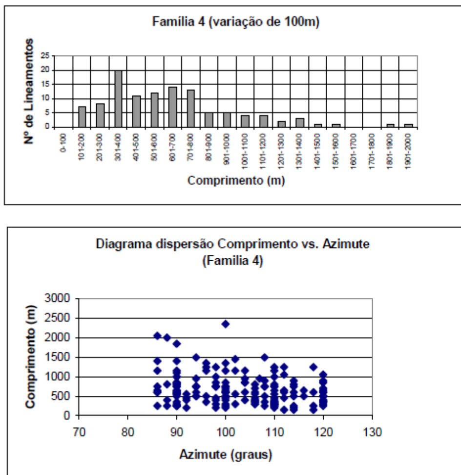
Figura 8 Histograma e diagrama de dispersão Família 4.
