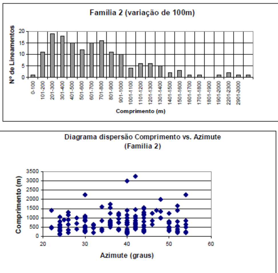
Figura 6 Histograma e diagrama de dispersão Família 2
