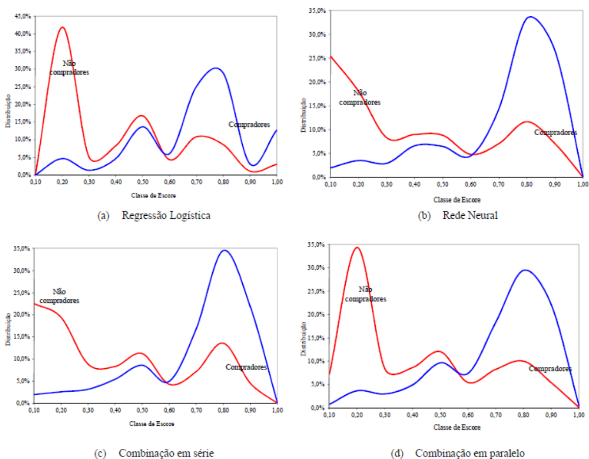
Figura 4 - Distribuição de compradores e não compradores por classe de score
