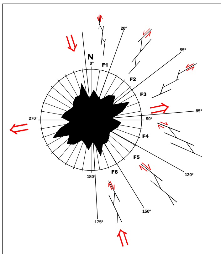
Figura 11 Padrões de ramificações desenvolvidos em cada família. As setas grandes indicam o campo tensional, segundo Reginato (2003), para áreas próximas.
