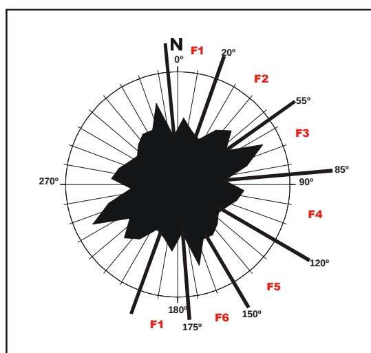
Figura 4 Histograma circular de frequência dos lineamentos tipo 2 – Bacia do Rio Três Forquilhas (862 medidas).
